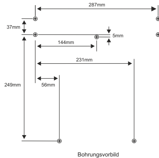
Bohrungsvorbild
